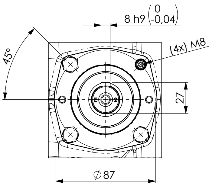
Detailed flange view Vista dettagliata flangia
