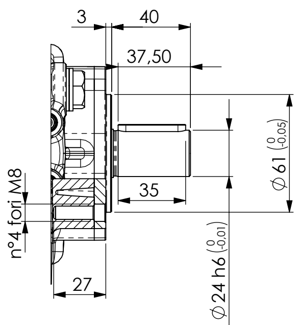
Detailed shaft view Vista dettagliata albero
